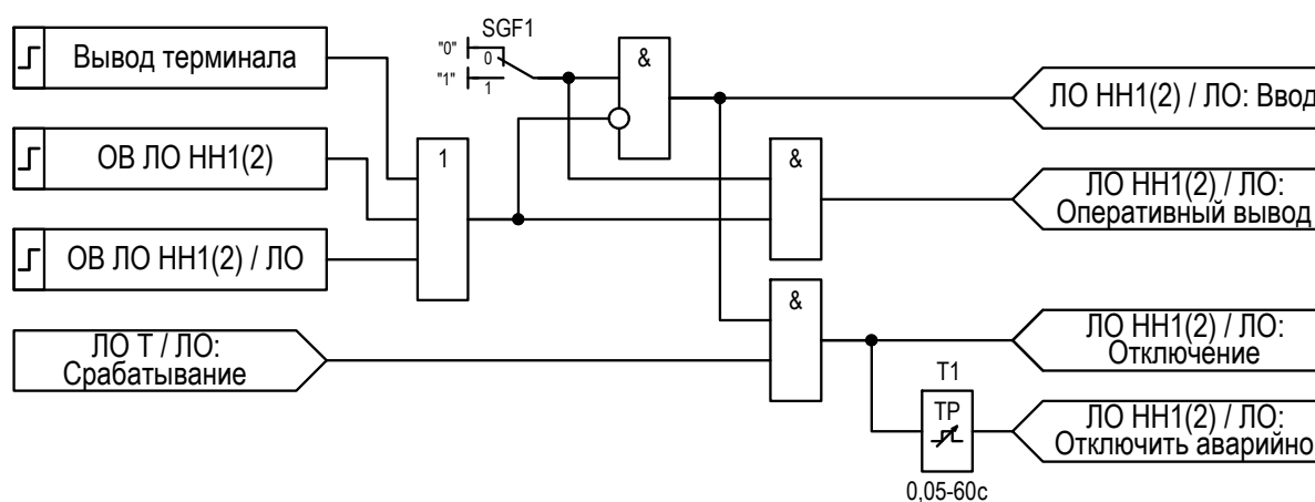
Рисунок 2.29 – Функциональная схема «ЛО»
