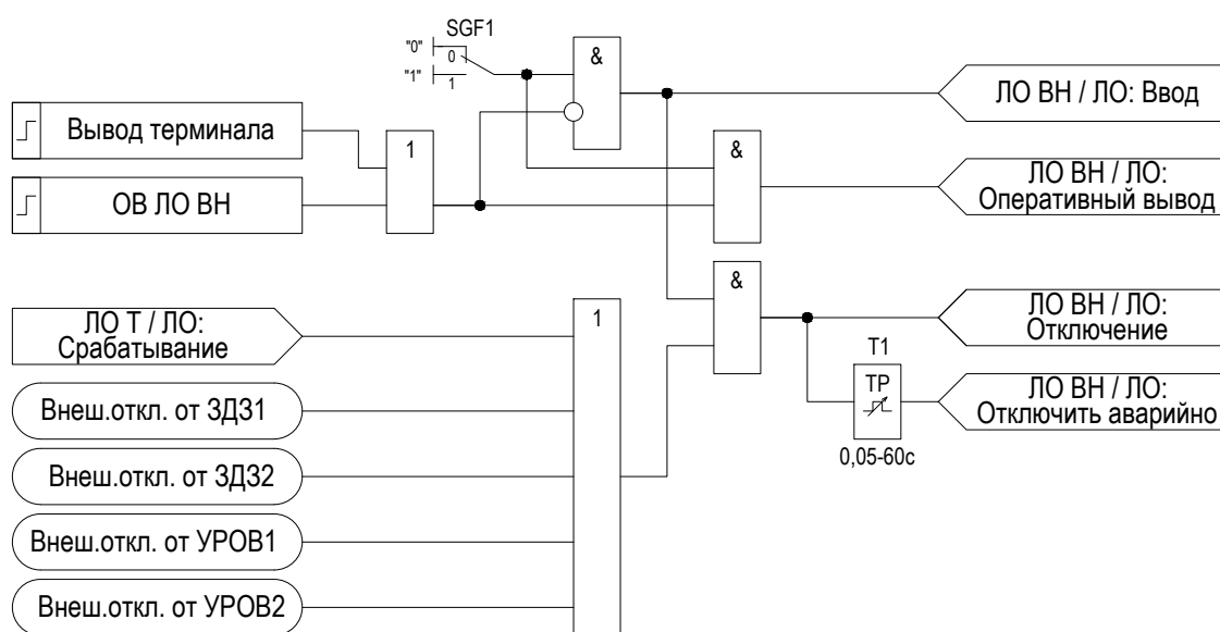
Рисунок 2.28 – Функциональная схема «ЛО»
